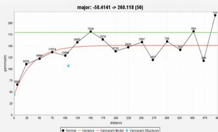
شکل پنجم واریوگرام دیتاهای آهن در جهت اصلی به همراه مدل رسم شده.
