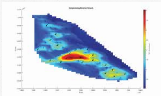
شکل ۱۱ شبکه ۲۰ برمه تکمیلی براساس تابع GET معیاری در بین شبکه اولیه حفاری
