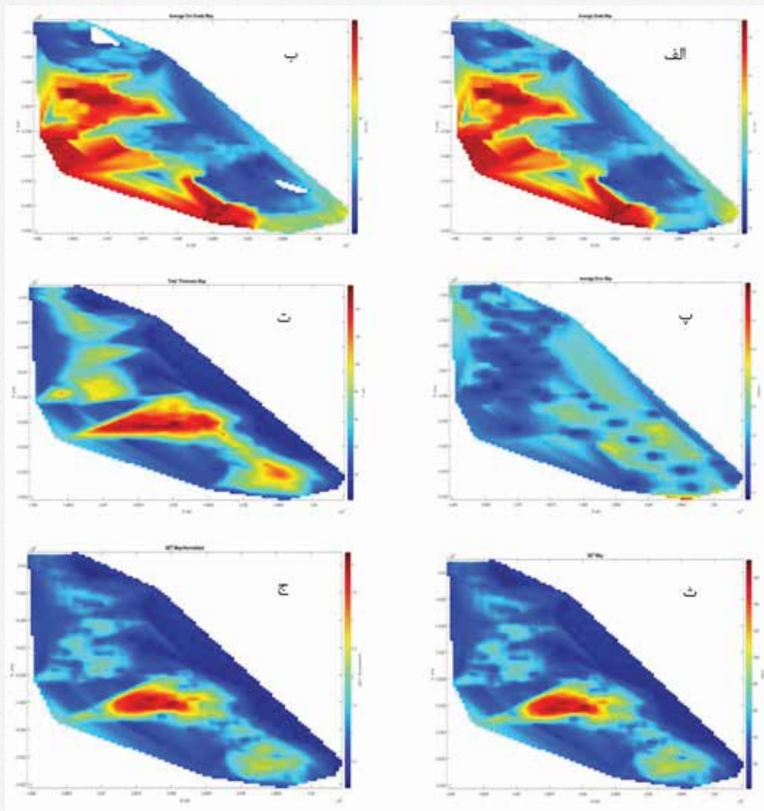
شکل هفت الف) نقشه عیار متوسط آهن، ب) نقشه عیار متوسط آهن با حداقل عیار (۲۰) فیصد، پ) نقشه خطای متوسط آهن، ت) نقشه مجموع ضخامت آهن، ث) نقشه تابع get و ج) نقشه تابع (GET) نرمال شده را نشان می‌دهد.
