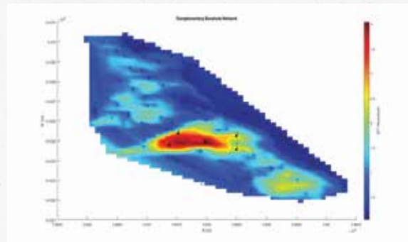
شکل هشت شبکه پنج برمه تکمیلی براساس تابع GET معیاری در بین شبکه اولیه حفاری
