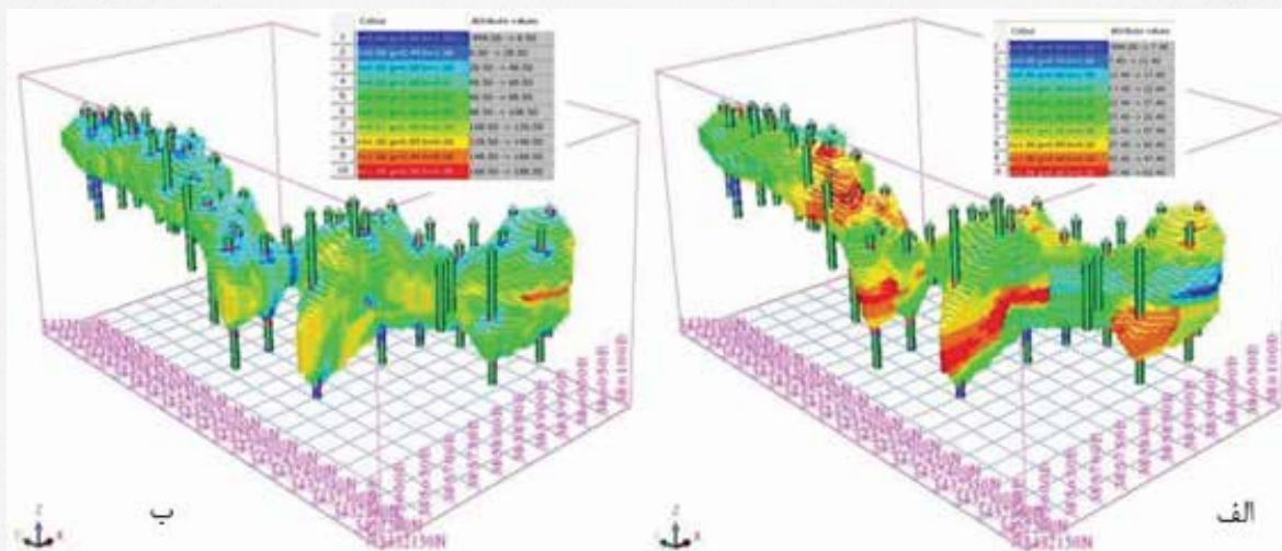
شکل شش مدل تخمینی سه بعدی بر اساس حداقل عیار (۲۰) فیصد، الف) توزیع عیار آهن، ب) توزیع واریانس آهن.
