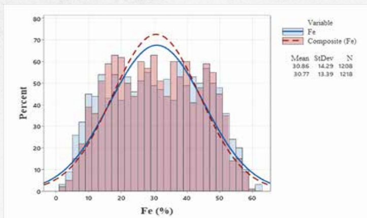
شکل چهار مقایسه دیتاهای خام و کامپوزیت م آهن بر اساس پارامترهای میانگین و انحراف معیار.
