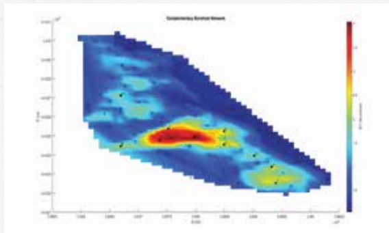
شکل نه شبکه ده برمه تکمیلی براساس تابع GET معیاری در بین شبکه اولیه حفاری
